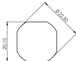
Otwór montażowy
