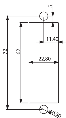
Otwór montażowy
