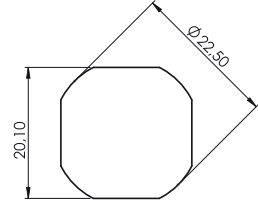
Otwór montażowy
