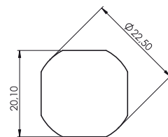
Otwór montażowy
