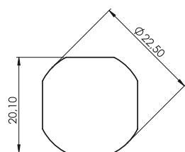
Otwór montażowy
